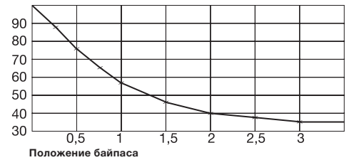
Расход теплоносителя для радиатора в %
